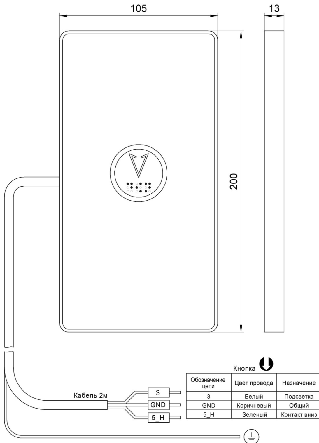
Рис.1 Внешний вид и габаритные размеры Вызывного поста МАЛАХИТ НШЕК.468381.083
